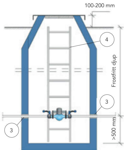
Figur 2: Sektion nedstigningsbar brunn.
